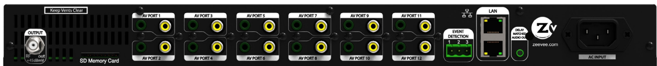
Coax Output AV Ports 10/100 LAN Ports Analog Audio Output AC Power Input
